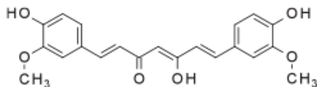
图二. 姜黄素的化学结构
